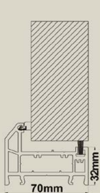
Low PVCu
